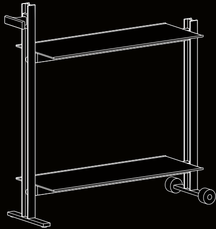
TROLLEY W74,5 CM D24 CM H77,5 CM
